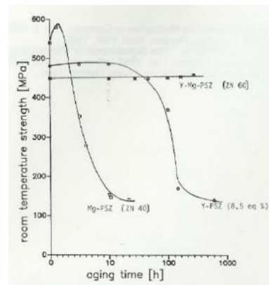
Figure 11. Thermal stability of Y-Mg-PSZ vs. Mg-PSZ.
